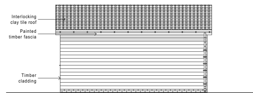
1:100 Elevation
